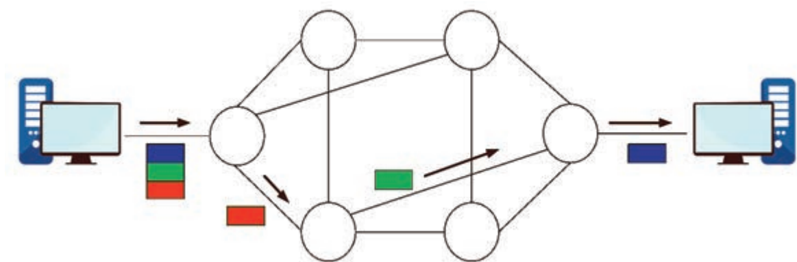
图 2.1.4 虚电路交换
