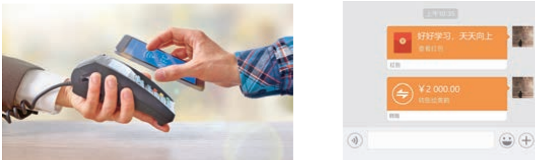
图4.2.2 移动支付
