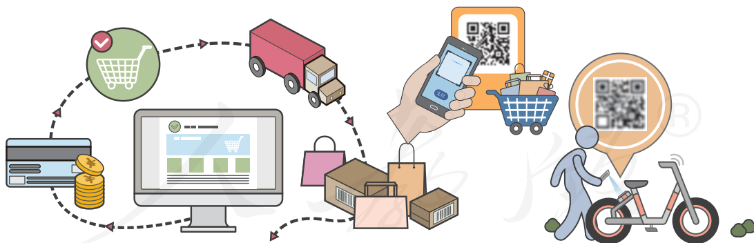
图4.2.1 网络应用
