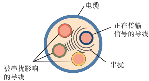
图 1.2.21 串扰示意图
