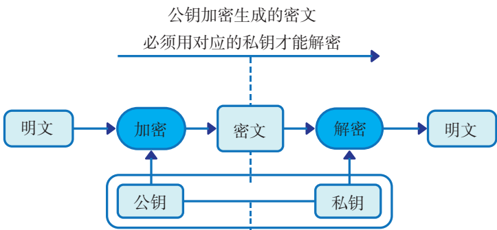
图 3.1.20 加密与解密
