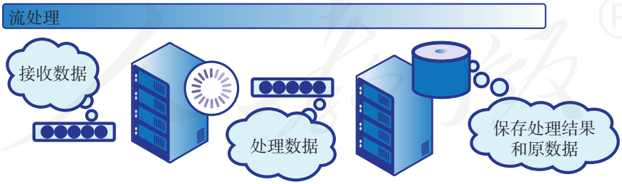
图 4.1.13 流处理
