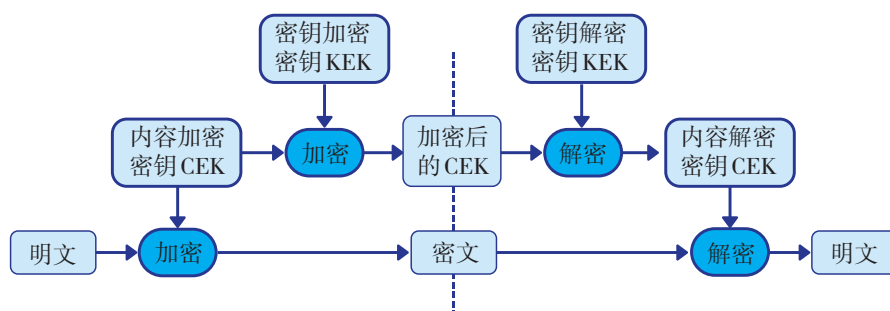
图 3.1.40 CEK 与 KEK
