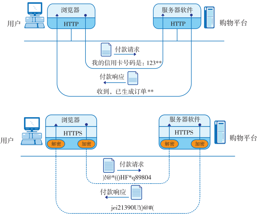
图 3.1.23 HTTP 与 HTTPS
