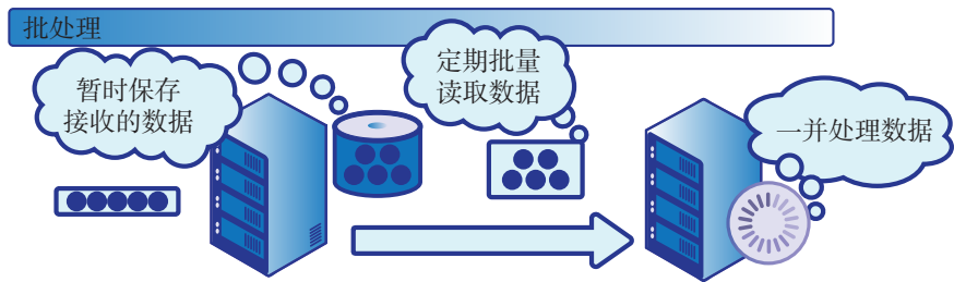
图 4.1.12 批处理
