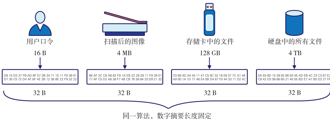
图 3.1.2 数字摘要
