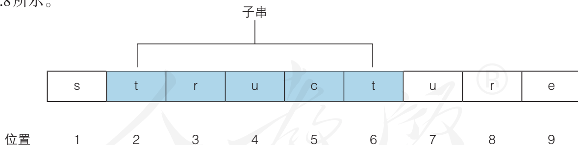
图3.4.8 获取子串
