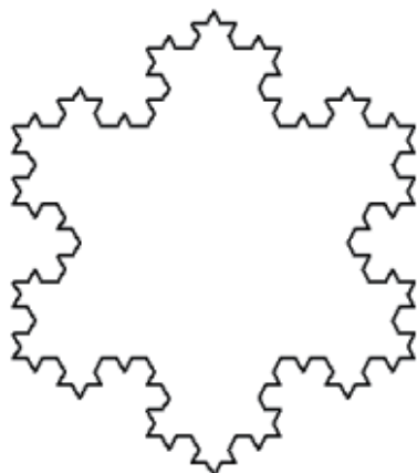
图4.3.7 雪花曲线
