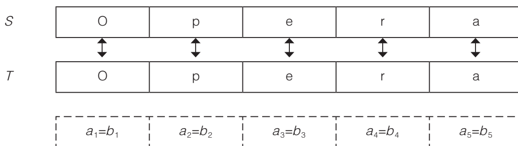
图 3.4.4 字符串比较 (1)
