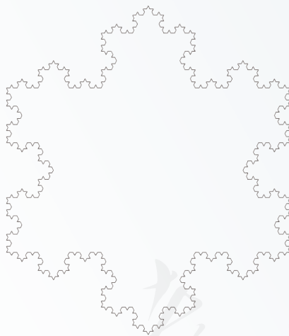
图4.3.9 4阶雪花曲线
