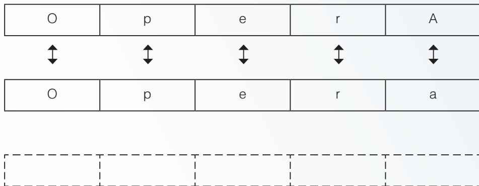
图3.4.7 字符串比较（4）
