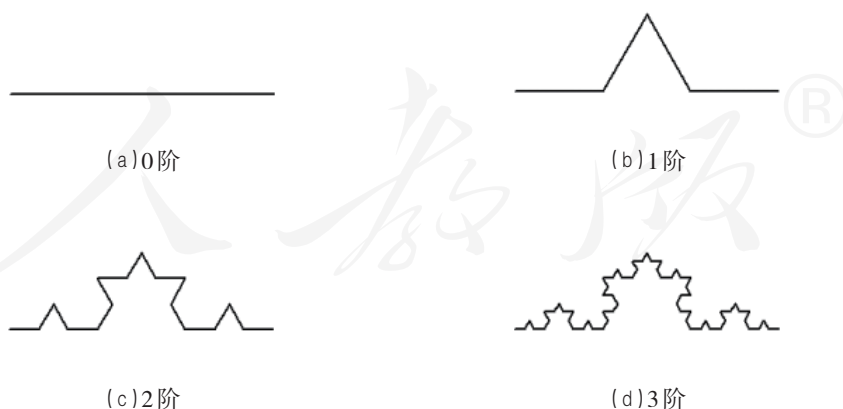
图4.3.8 单边的雪花曲线
