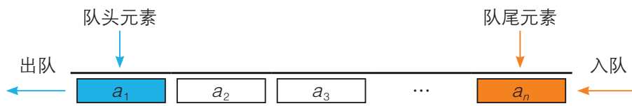
图3.3.4 队列示意图
