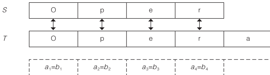
图 3.4.5 字符串比较 (2)
