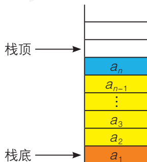
图3.2.4 栈的示意图
