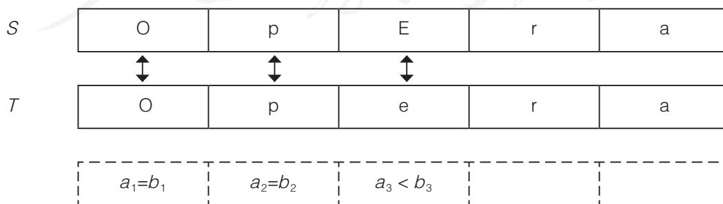
图 3.4.6 字符串比较 (3)
