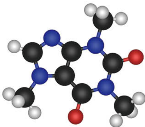
咖啡因分子结构图
