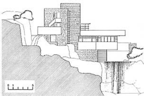
西立面图
