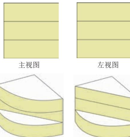
根据图中的主视图和左视图，再画出两个以上的立体图。
