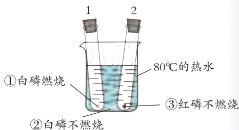
图3-43 燃烧实验
