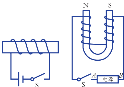
图1-27 通电螺线管
