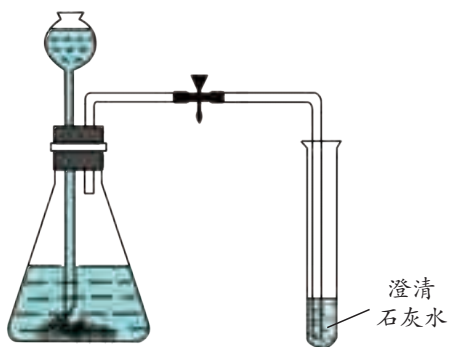
图3-60 \text{CO}_2 与澄清石灰水反应
