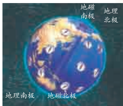
图1-14 地磁场
