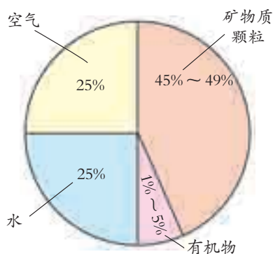
图4-14 壤土类土壤的组成 (按各成分体积分数的模型)
