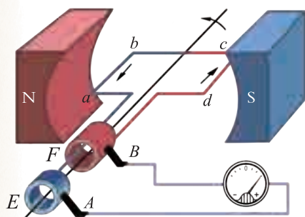
图1-51 交流发电机的原理
