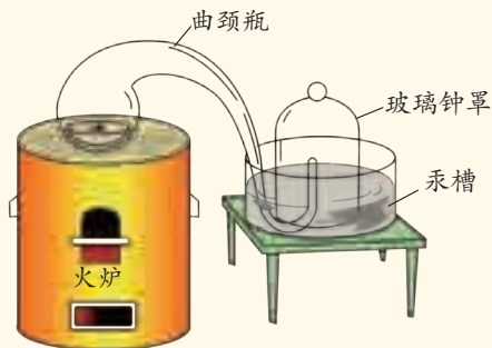
图3-17 拉瓦锡研究空气成分所用的装置
