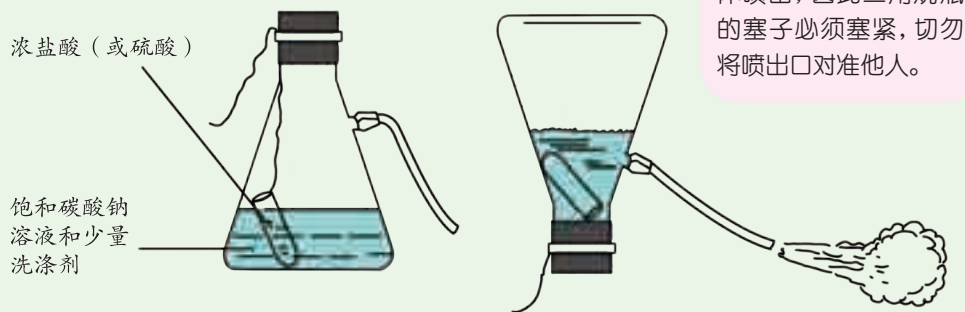
图3-63 简易酸碱灭火器
