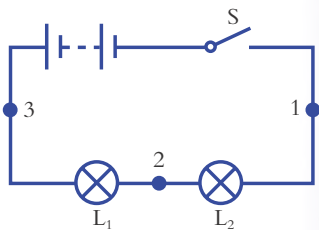
图4-24 串联电路图
