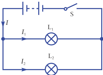
图4-55 电路图2
