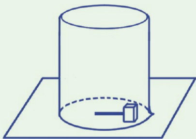
图2-4 对流实验
