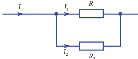
图4-66 电路图
