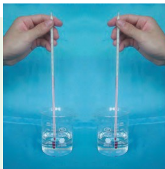
图1-42 溶解的吸热与放热实验
