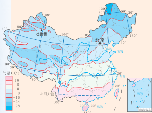
图2-51 我国1、7月份平均气温分布图
