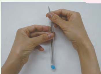
图1-39 固体药品的取用
