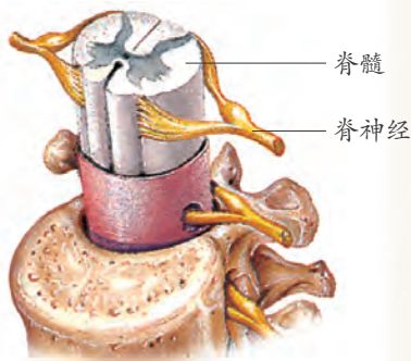
图3-17 脊髓剖面图
