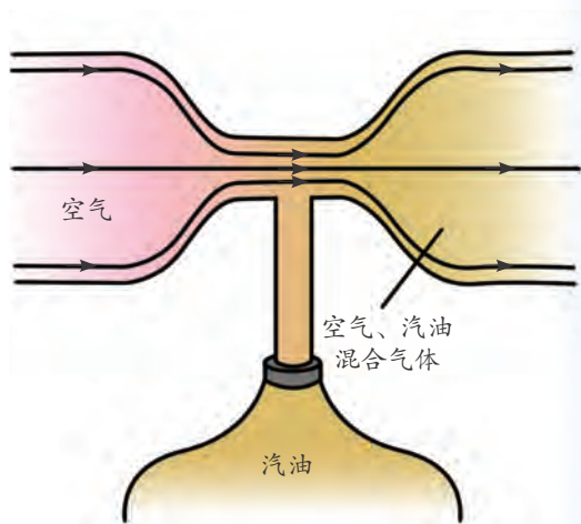
图2-33 化油器示意图
