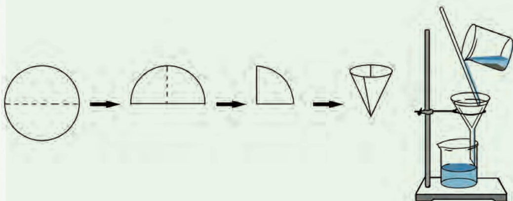
图1-52 过滤泥浆水
