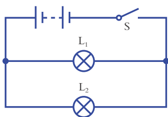
图4-27 电路图
