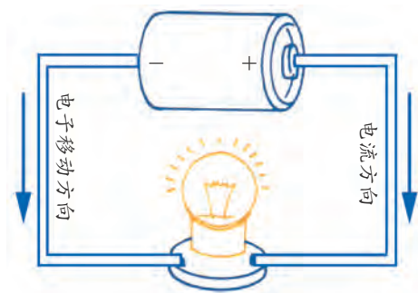
图4-8 电流方向和电子运动方向
