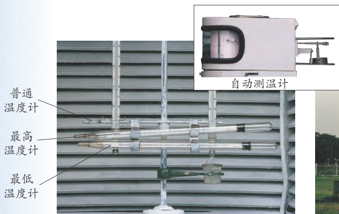
图2-7 最高温度计和最低温度计
