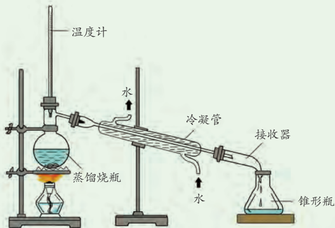
图1-53 蒸馏装置
