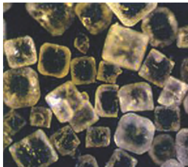
食盐晶体
