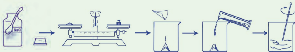
图1-45 配制一定溶质质量分数的溶液的步骤示意图
