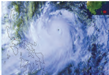
图2-63 台风
