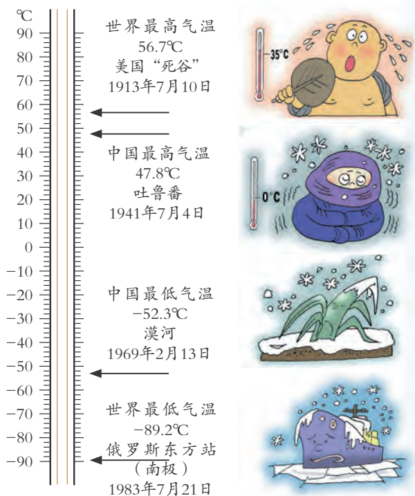
图2-10 气温与人们的生活
