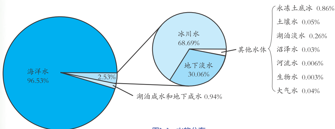
图1-1 水的分布
