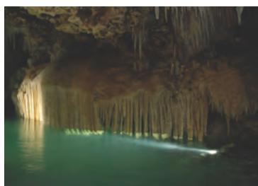
神秘莫测的地下暗河
