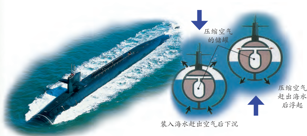
图1-27 潜艇
