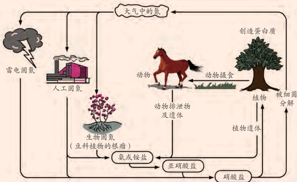
图2-28 氮的循环
