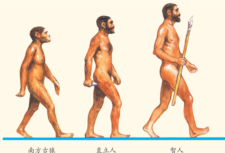
图1-43 人类的进化
