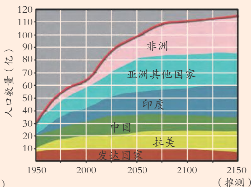
图4-2 人口增长
