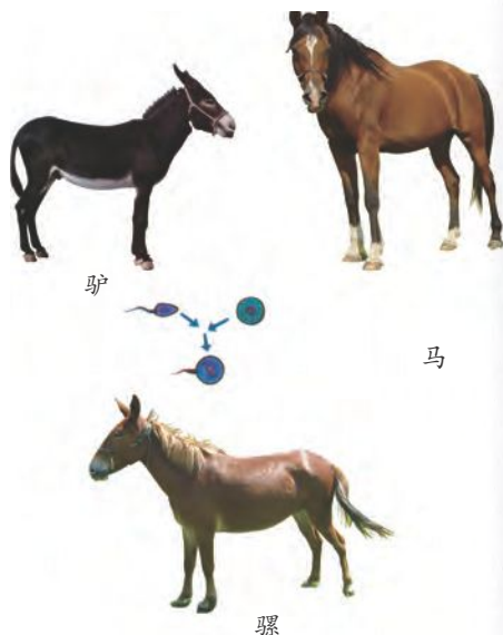
图1-50 杂交优势
