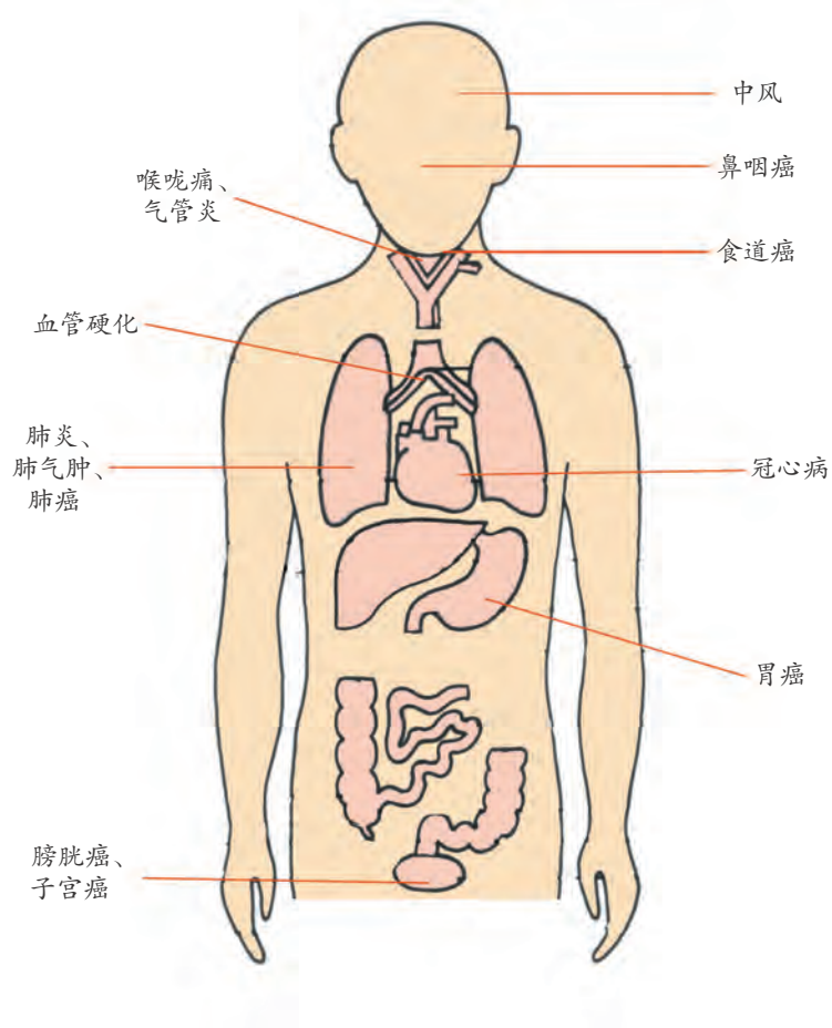
图3-36 香烟的危害
