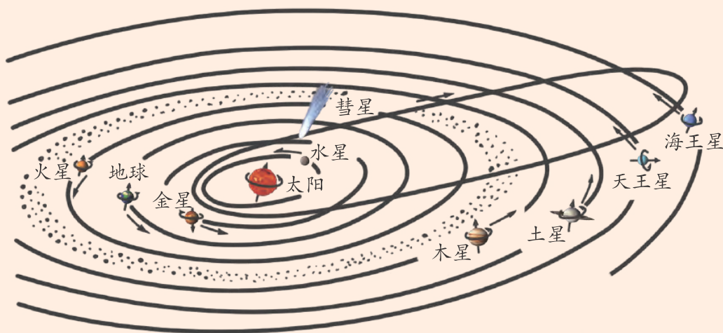
图1-10 太阳系
