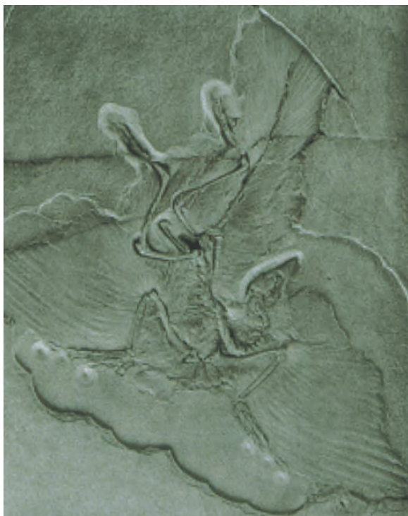
图1-38 始祖鸟化石
