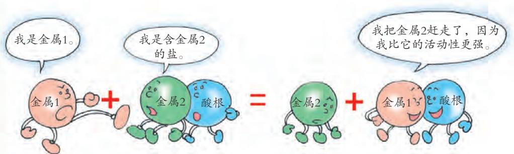
图2-15 置换反应示意图
