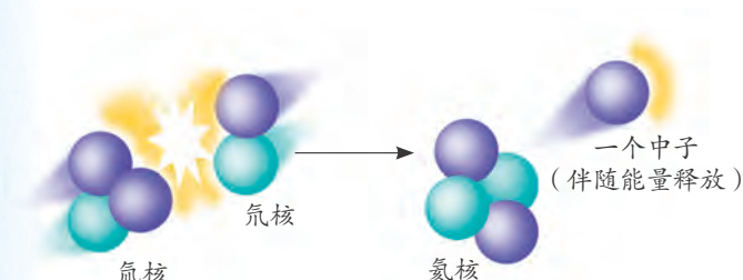
图3-89 聚变反应示意图
