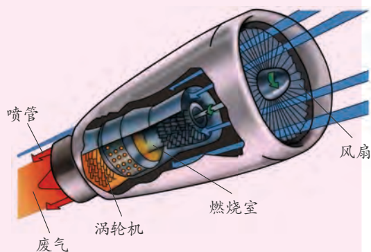
图3-71 空气喷气发动机
