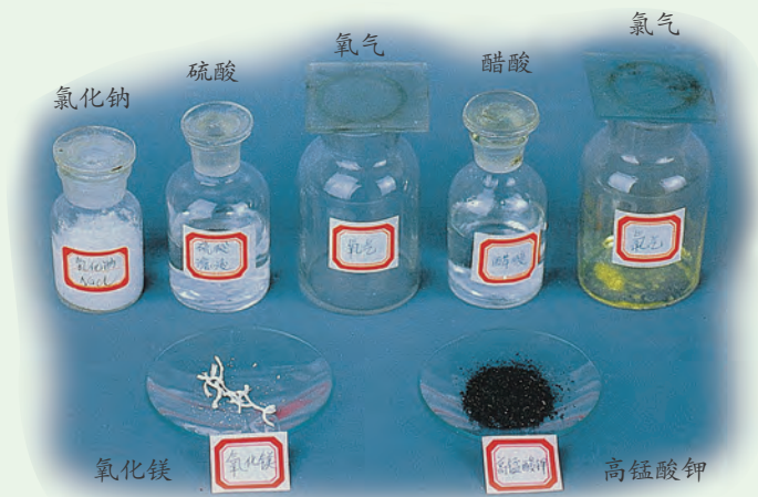
图2-32 7种不同的物质
