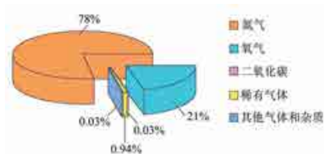
图3-1-3 空气中各成分含量(体积分数)示意图
