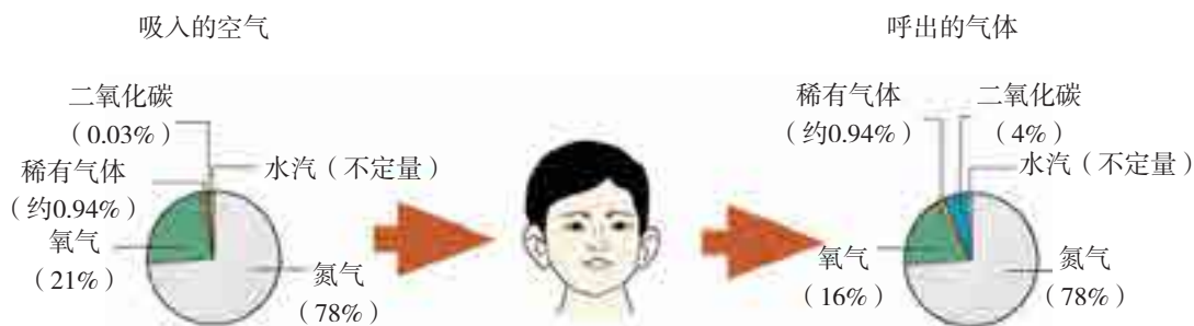
图5-1-2 吸入的空气与呼出的气体成分比较
