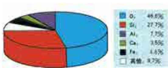
图6-2-4 地壳中的元素含量分布
