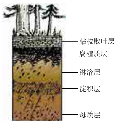
图9-5-2 我国东北的灰化土层次
