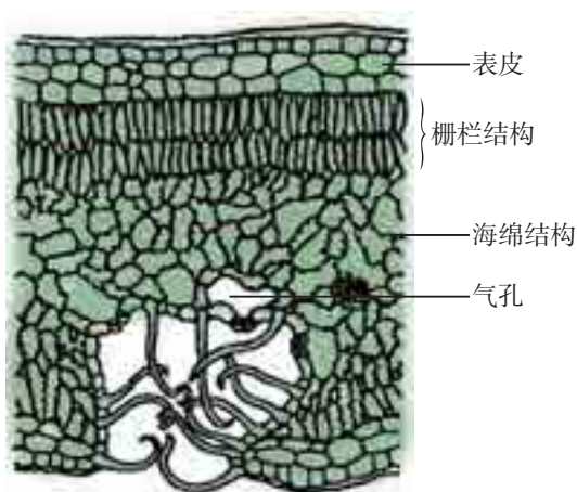
图4-3-4 夹竹桃叶横切面示意图
