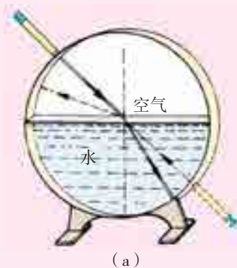
图9-3-2 光的折射
