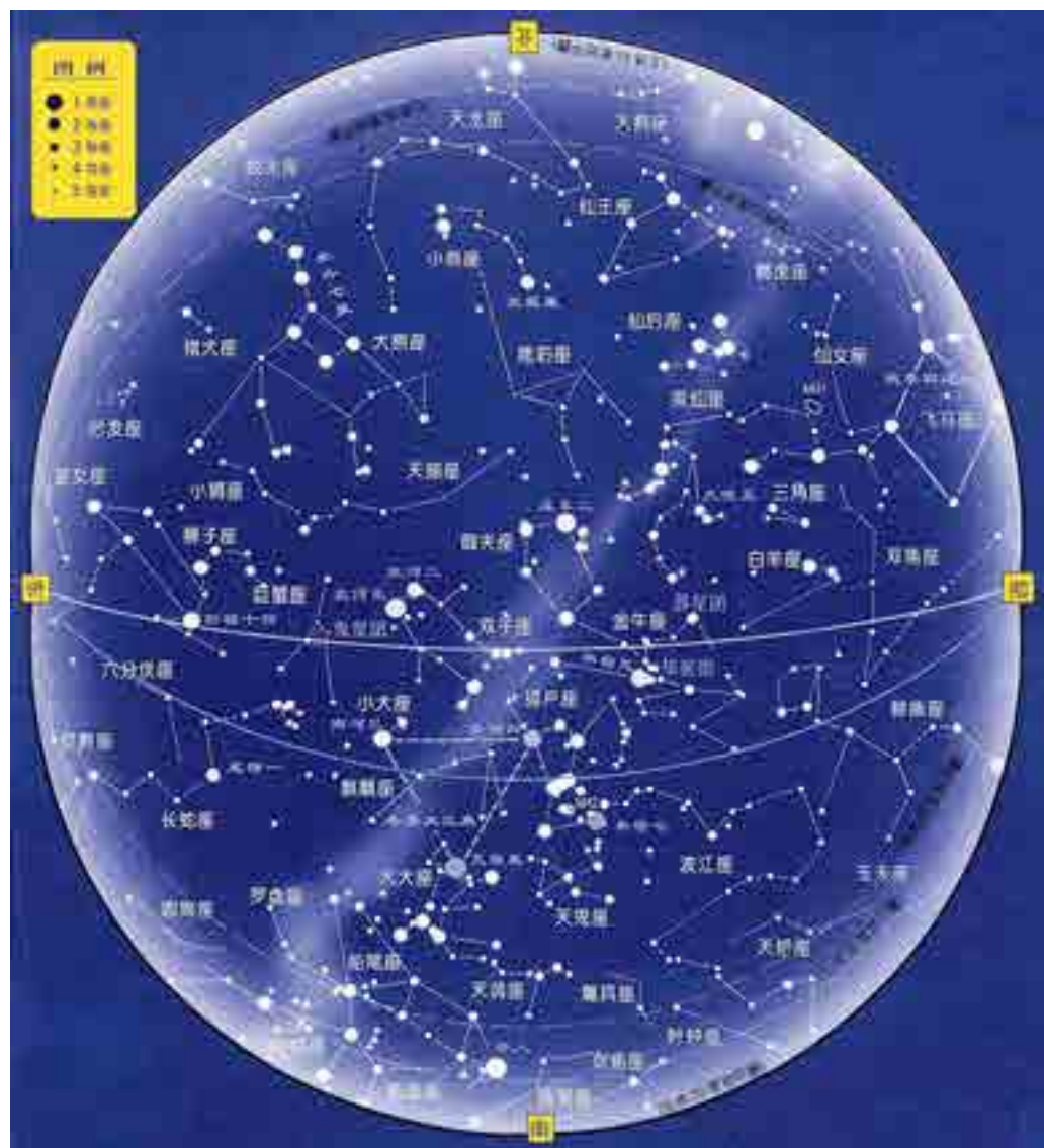
图7-3-4 冬季星空
