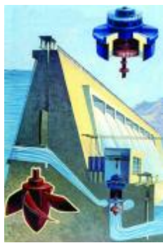
图 2.1 堤坝式水电站示意图
