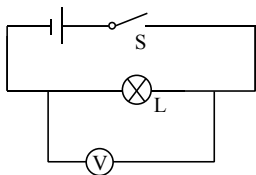
图 4.36 电压表的接入电路图
