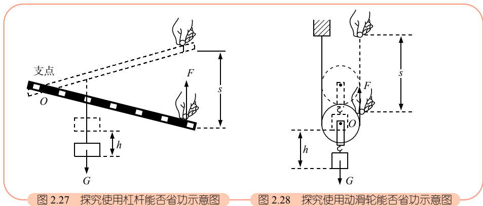
图 2.27 探究使用杠杆能否省功示意图
