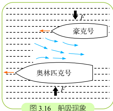
图 3.16 船吸现象
