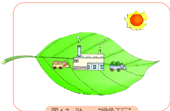
图 6.7 叶——“绿色工厂”
