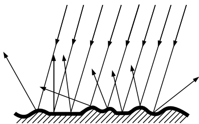
图 1.37 漫反射
