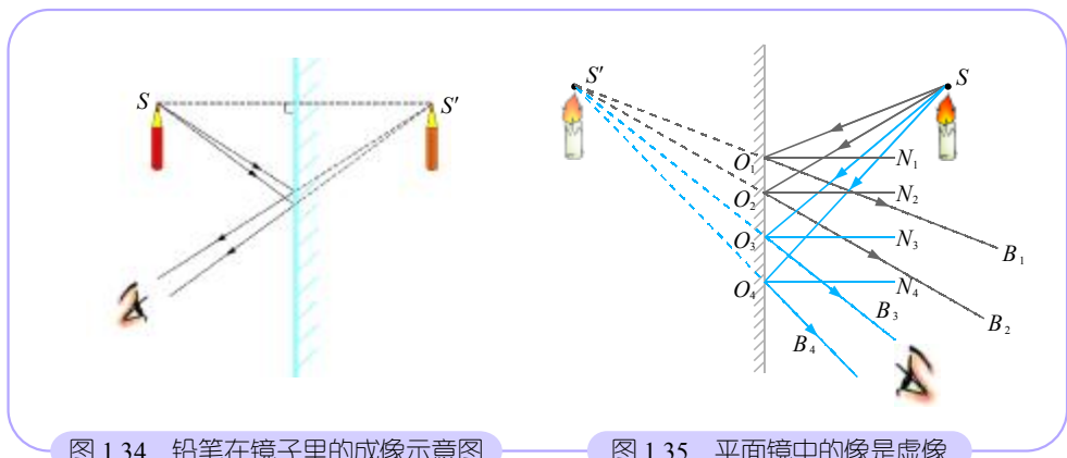
图 1.34 铅笔在镜子里的成像示意图
