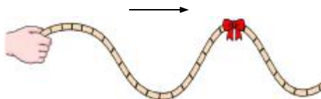
图 1.13 沿绳传播的波
