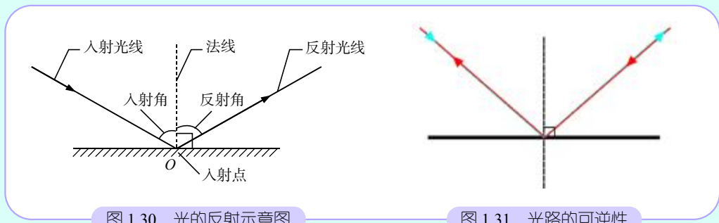
图 1.30 光的反射示意图
