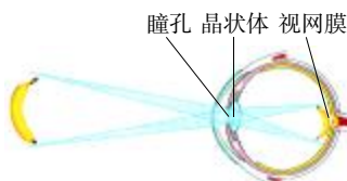
图 1.45 人眼的成像示意图
