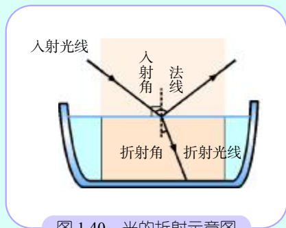
图 1.40 光的折射示意图
