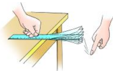
图 1.9 乐音的响度与音调实验
