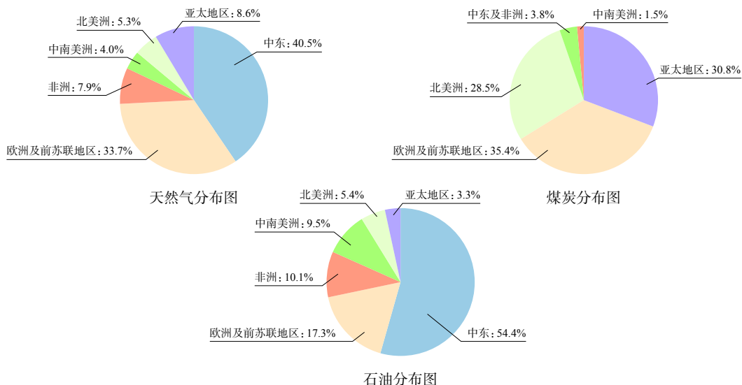
图 4.4 2010 年世界石油、天然气和煤炭储量地区分布图
