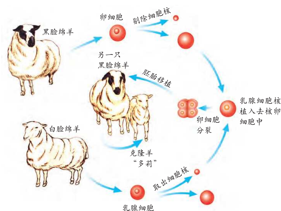
图 7.2-9 “多莉”的培育过程示意图
