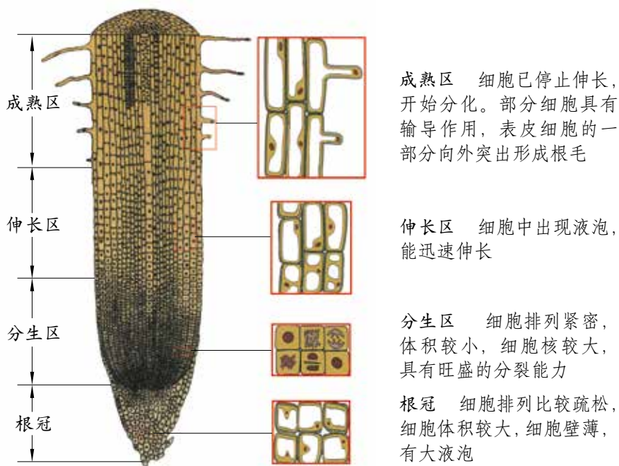
图 4.1-26 根尖的结构示意图
