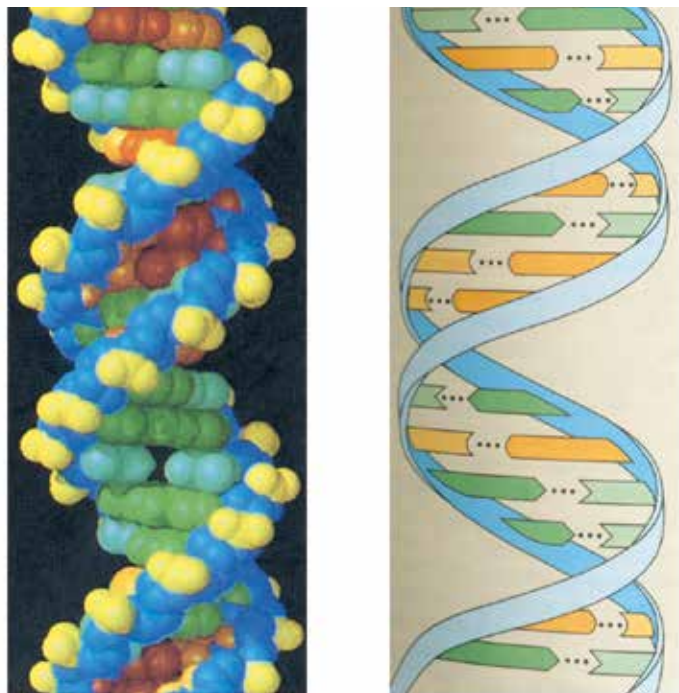
图 4.4-3 DNA 分子模型(左)和双螺旋结构示意图(右)
