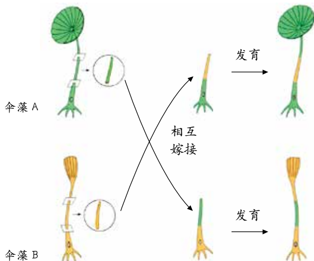
图 4.4-1 伞藻嫁接实验
