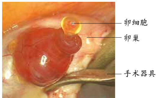
图 4.3-5 正在排出的卵细胞(50×)
