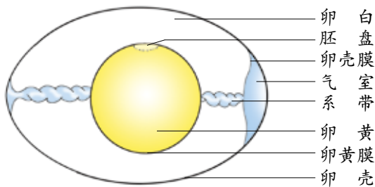
图 4.2-24 鸟卵结构示意图
