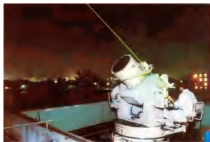
图 3-29 用于测控人造卫星的固定式激光测距仪
