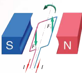
(c) 通电线圈越过平衡位置后,磁场力会使它逆时针旋转
