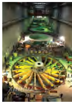
图 16-40 水轮发电机组
