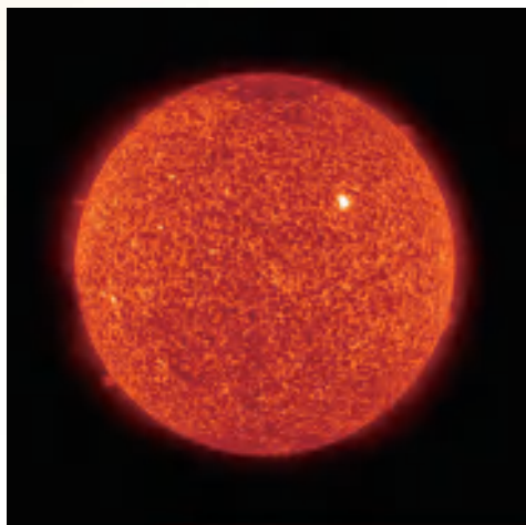
图 18-31 太阳
