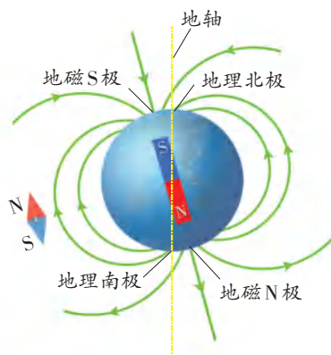
图16-8 地磁场
