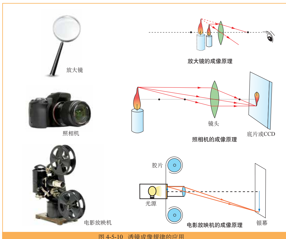
图 4-5-10 透镜成像规律的应用
