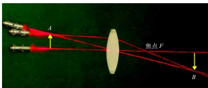
图 4-5-9 用几束光探究透镜成像的规律
