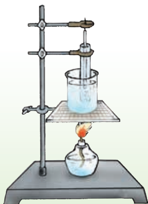
图5-2-6 研究熔化现象的实验装置
