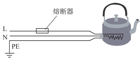
图 9-1-4 电水壶接电路示意图
