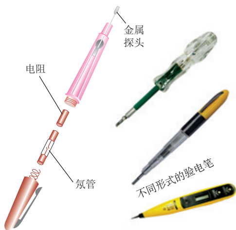
图 9-1-7 常见的验电笔前端为金属探头,后端为金属挂钩或金属片,中间绝缘管内装有发光氖管、电阻及压紧弹簧
