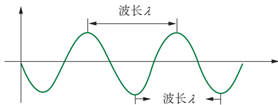
图 10-1-4 波的图像
