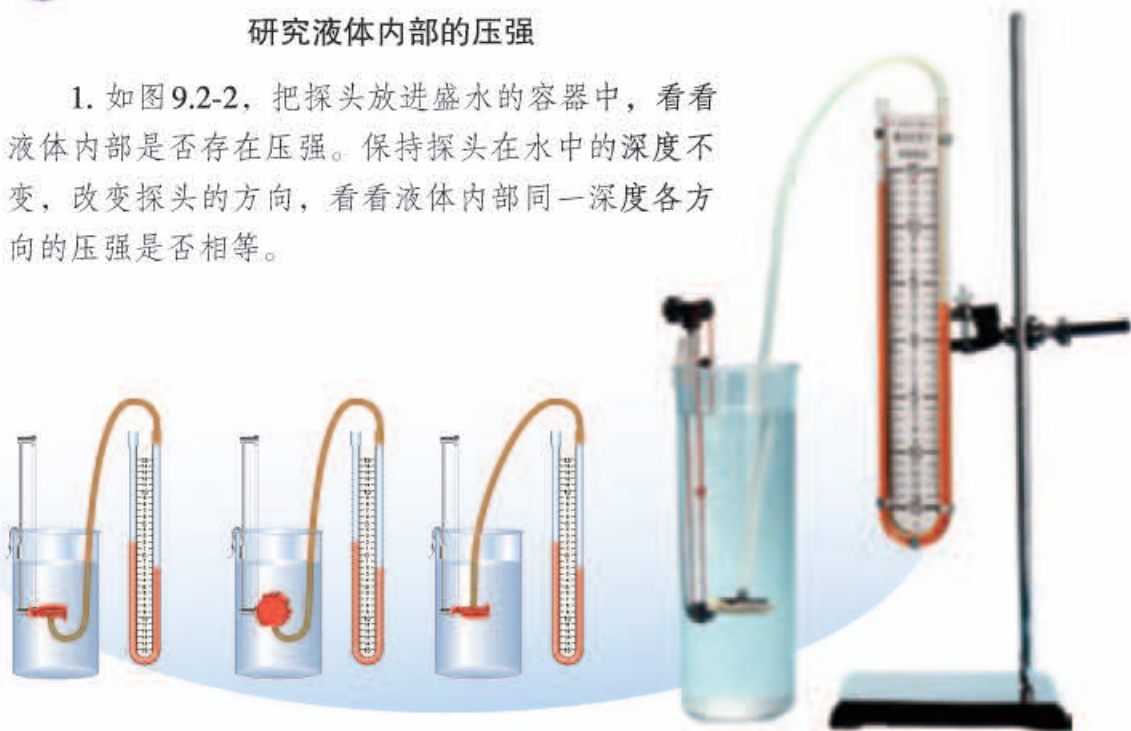
图9.2-2 同一深度液体向各个方向的压强是否相等?
