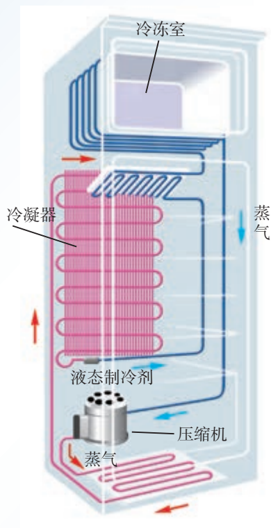
图3.3-8 电冰箱原理图
