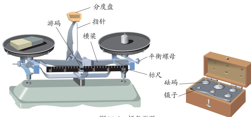
图6.1-2 托盘天平
