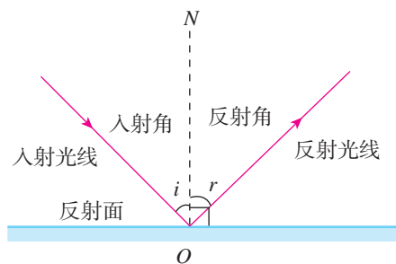
图4.2-4 光的反射
