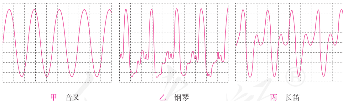
图2.2-4 声音波形图
