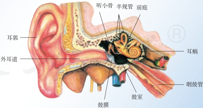
图2.1-8 人耳构造
