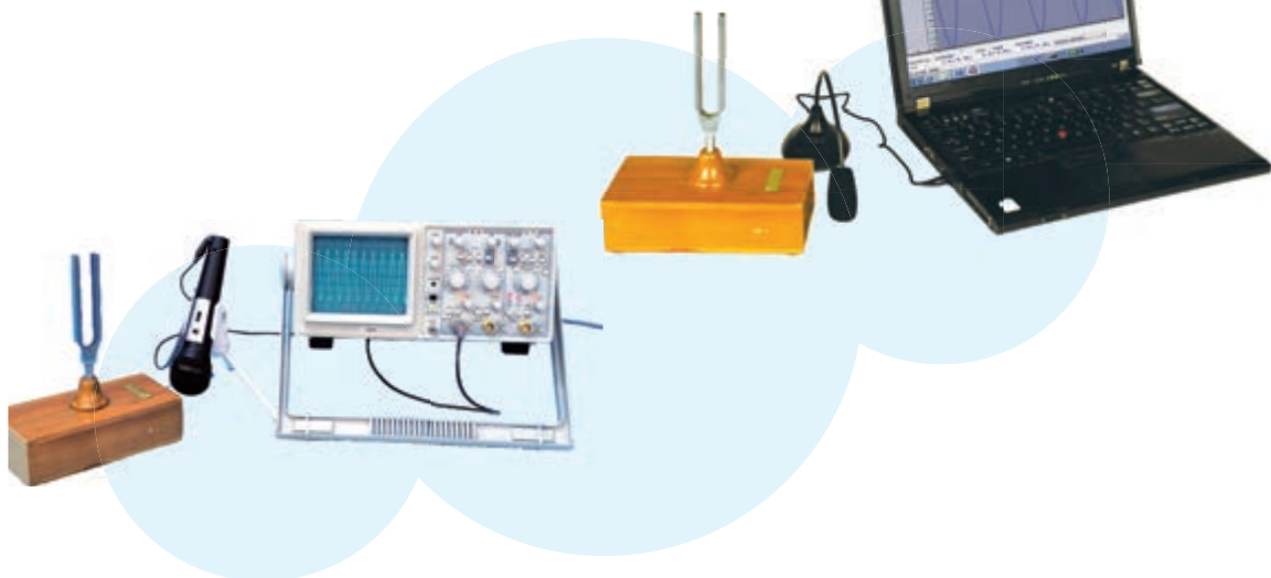
图2.2-2 声音的波形
