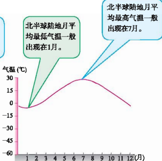
图 3-2-3 气温的年变化
