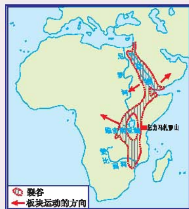
图 2-2-7 东非大裂谷
