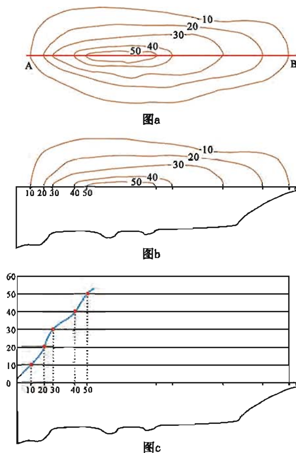
图 1-3-10 地形剖面图制作方法
