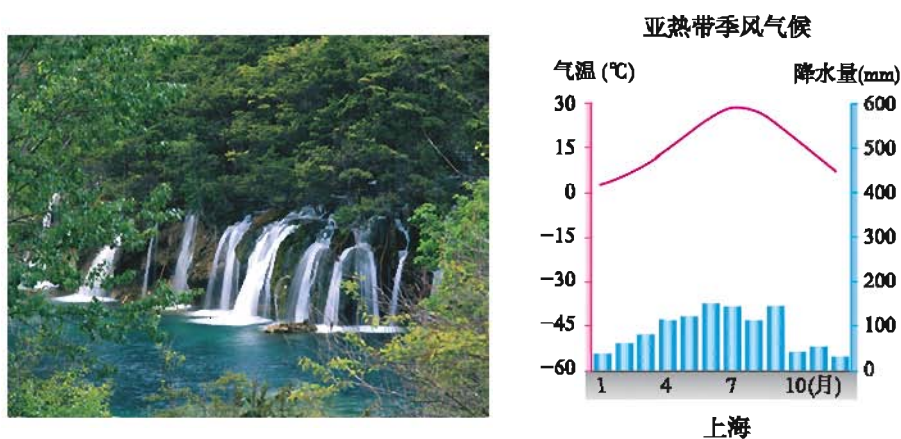
图 3-3-8 亚热带季风气候与自然景观
