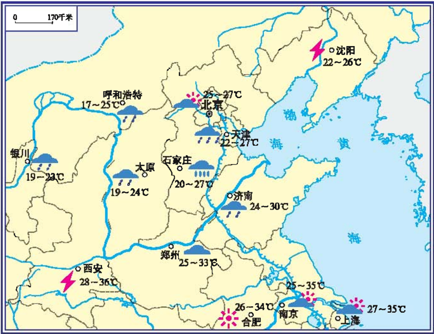
图 3-1-7 我国部分城市某日天气预报图
