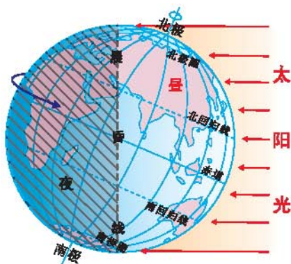
图 1-2-1 地球的自转
