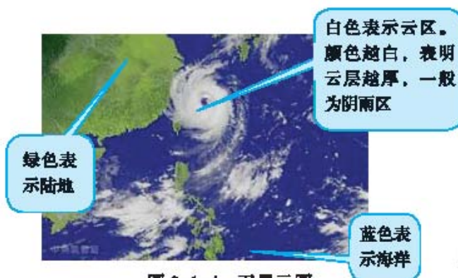
图 3-1-4 卫星云图
