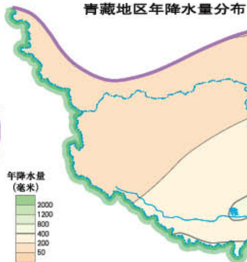
青藏地区年降水量分布
