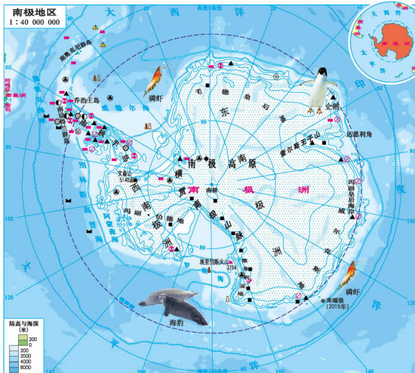
南极部分科学考察站
