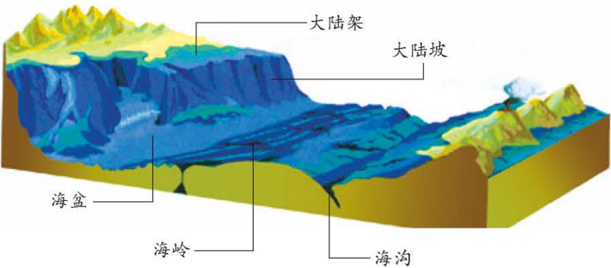
海底地形示意图
