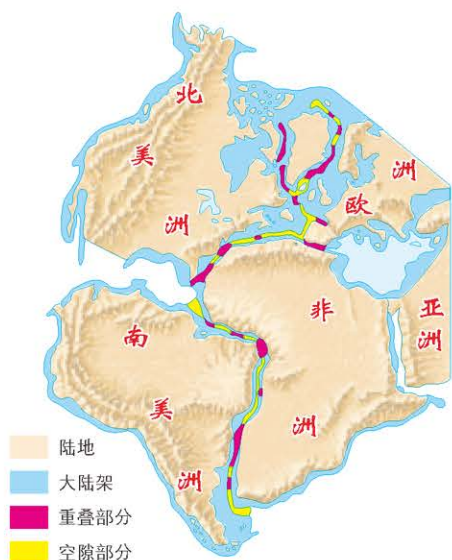
大西洋两侧陆块的拼合
