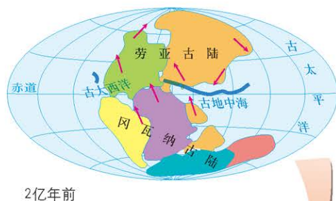
大陆漂移过程
