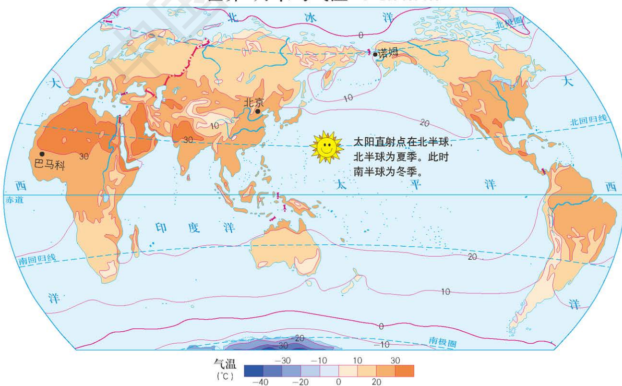
世界7月平均气温 1 : 200 000 000
