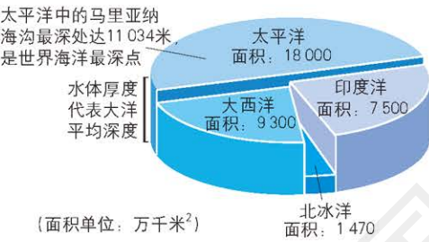
四大洋面积、海深的比较
