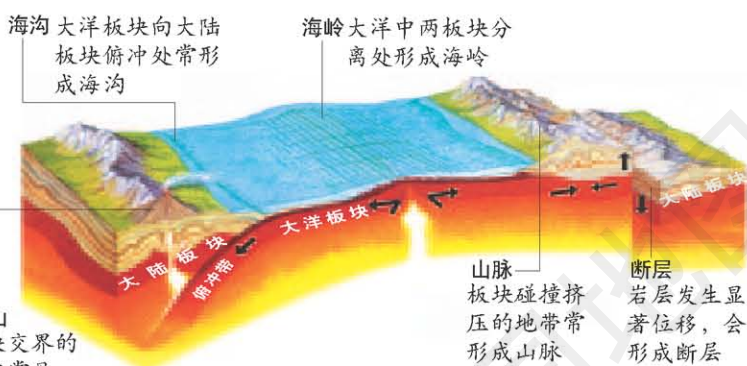
大洋板块俯冲示意
