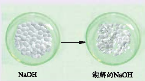
图7-14 固体氢氧化钠在空气中的潮解
