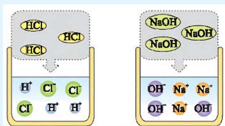
图7-7 HCl和NaOH溶解过程示意图
