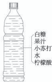
图9-20 自制汽水
