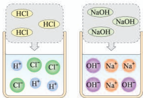
图 10-10 \text{HCl} 和 \text{NaOH} 在水中的解离出离子
