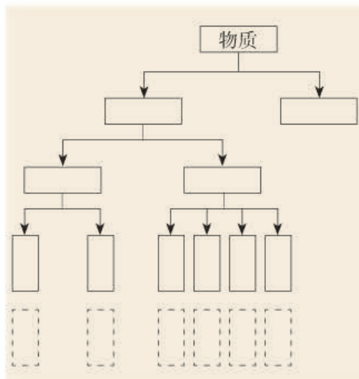
图 11-5 物质的分类
