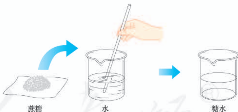
图9-2 蔗糖溶解
